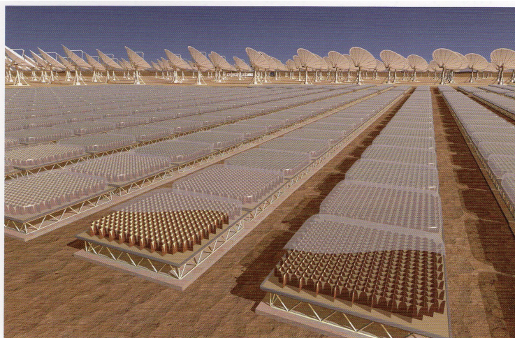
Fig. 2 – SKA (Square Kilometer Array) le radiotélescope du futur (image de synthèse). Projet mondial estimé à plus de 2 milliards d'Euros, il aura une surface collectrice d'un kilomètre carré. L'un de ses objectifs phares est de sonder l'Univers primordial dans une période où il n'a pas encore formé les premières galaxies. (SKA). ■
